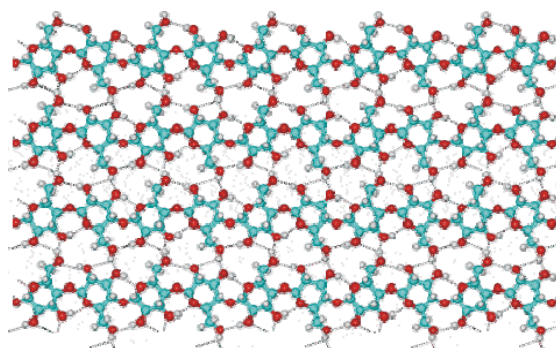
Gambar 1. Model molekul selulosa.
